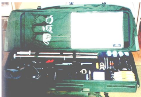
Podstawowe przenośne narzędzia wykorzystywane przez specjalistę pirotechnika
