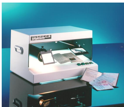
Podstawowe urządzenie do wstępnej kontroli autentyczności dokumentów paszportowych
