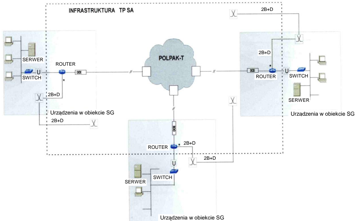
Rys. 3. Rozwiązanie szczegółowe fragmentu sieci na poziomie oddziału Straży Granicznej
